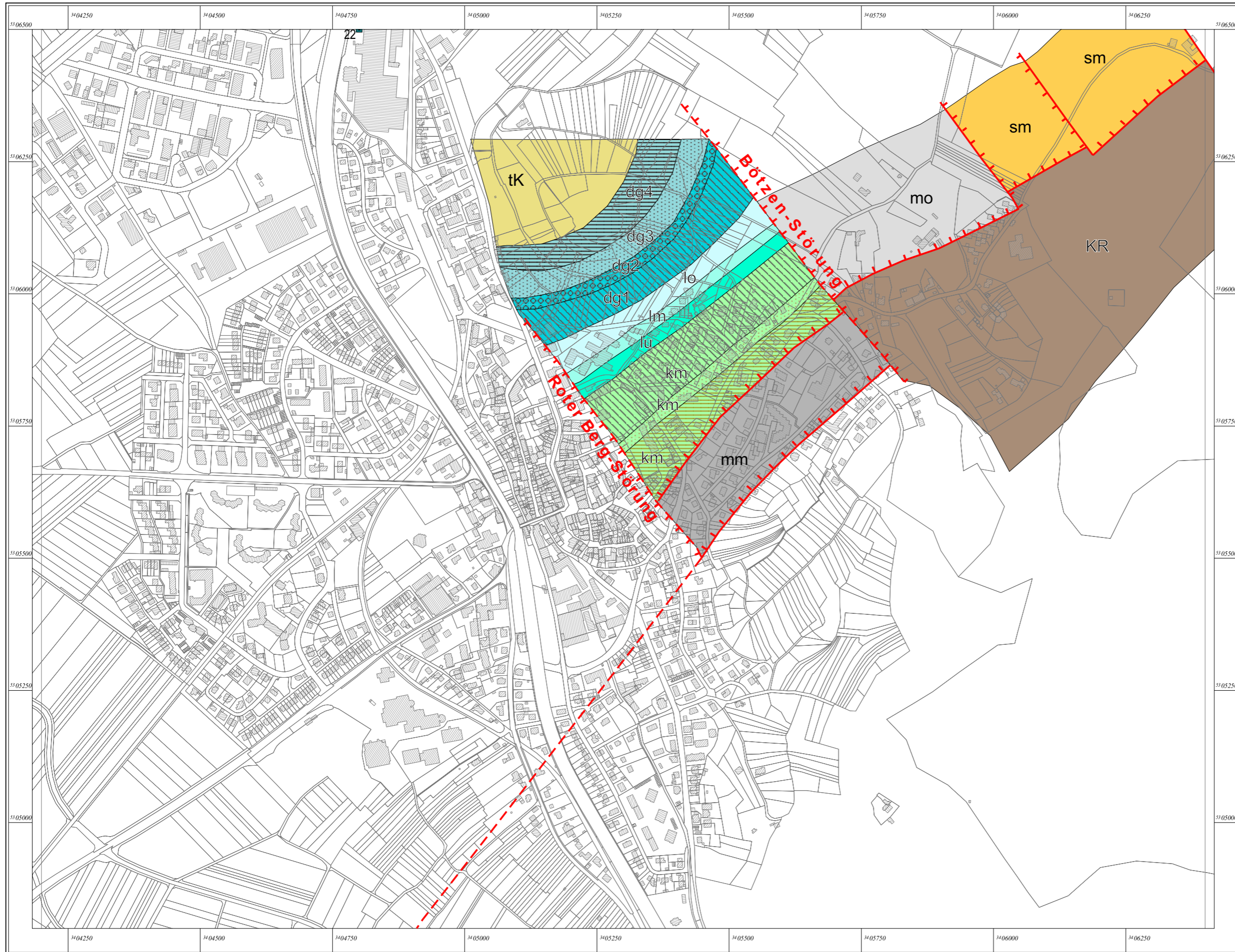
Geologische Karte nach GENSER (1959) (in Klammern: Abkürzung nach Symbolschlüssel Geologie RPF/LGRB Febr. 2010)
