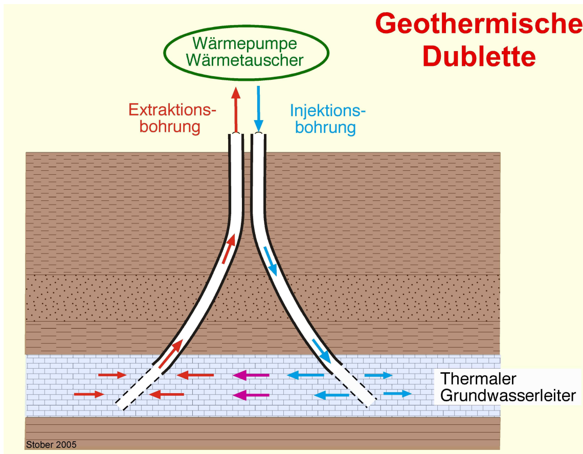
Abb. 2: Schema einer hydrothermalen Nutzung (Dublette)
