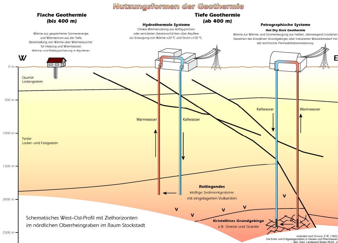
Abb. 1: Beispiele für Nutzungsformen der Geothermie
