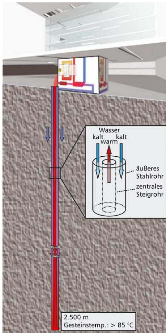
Abb. 5: Schema für eine tiefe Erdwärmesonde
