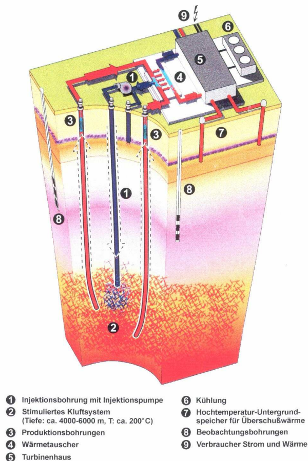
Abb. 4: Schema für ein HDR-Vorhaben
