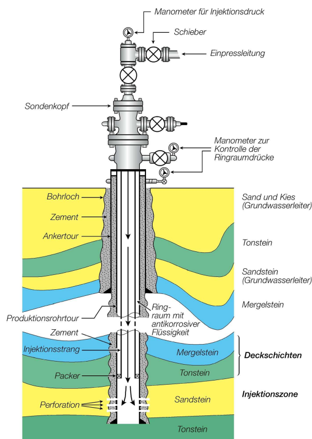
Abb. 3: Schema einer Injektionsbohrung
